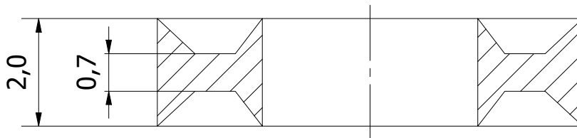
A-A ( 10: 1 )
