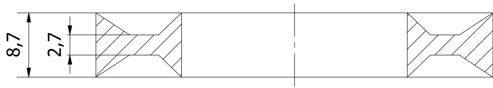
A-A ( 2 : 1 )
